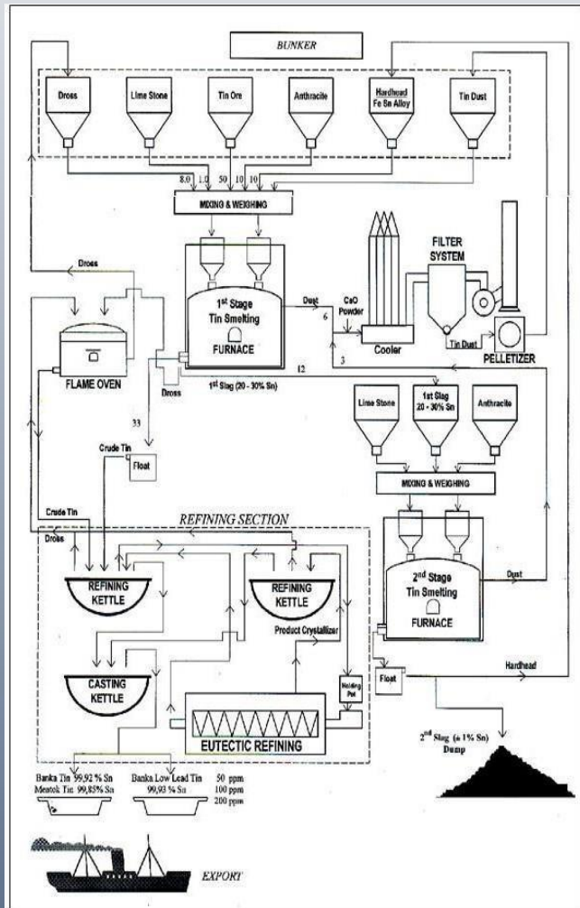
Gambar 13 Proses Produksi
