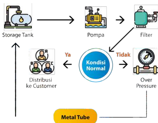
Gambar 5. Flow diagram setelah adanya metal tube
