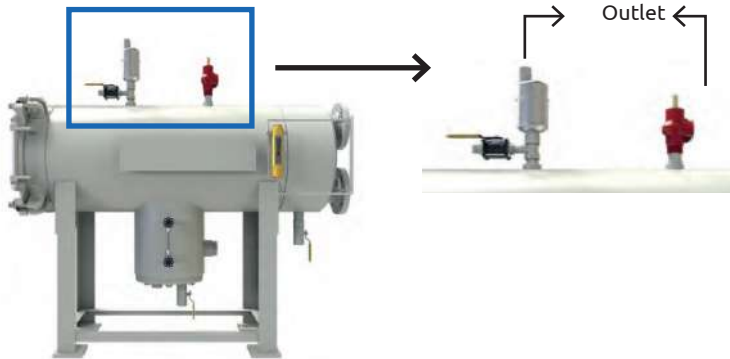
Gambar 3. Ilustrasi outlet air eliminator dan PSV
