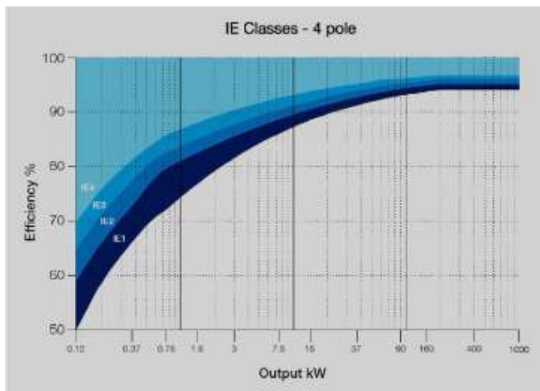
Gambar 2. Grafik Efisiensi Motor (%) Terhadap Daya Output Motor (kW)
