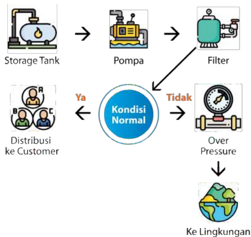
Gambar 4. Flow diagram sebelum adanya metal tube
