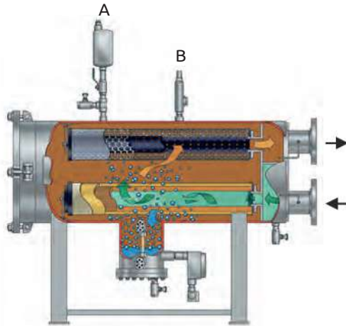
Gambar 1. Ilustrasi Posisi Air Eliminator (A) dan PSV (B) pada FWS
